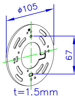
ボックス用プレート
