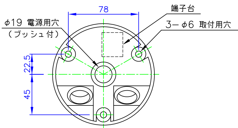
取付面図
