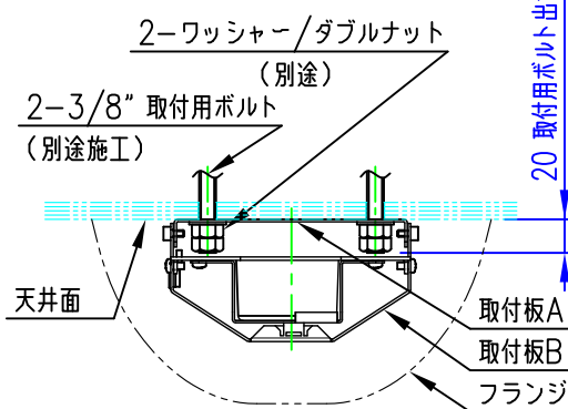
天井取付部詳細図
