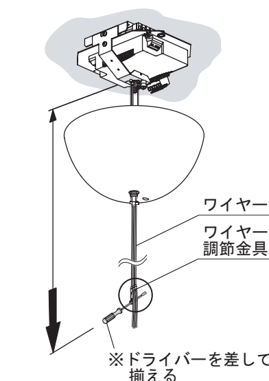
図2 ワイヤーの調整方法
