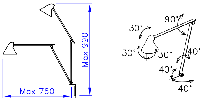
可動寸法および角度
