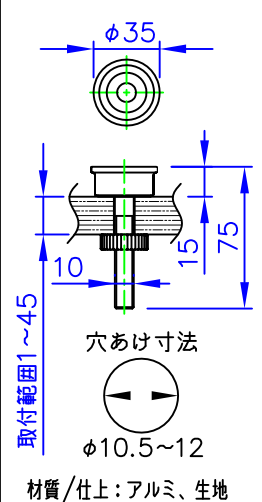
ピン寸法図
