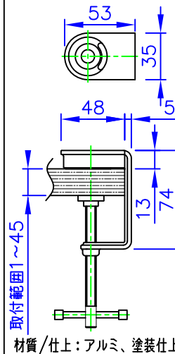
クランプ寸法図
