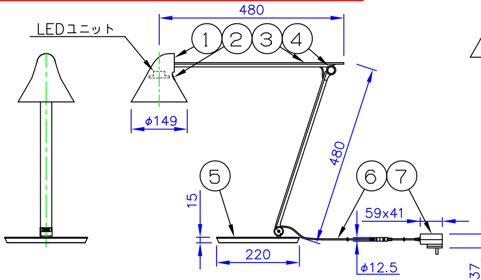
可動寸法および角度
