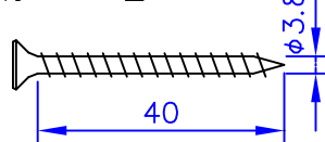
取付ネジ×2
