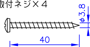
取付ネジ×4
