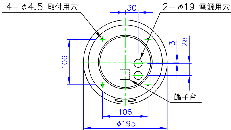
取付面図
