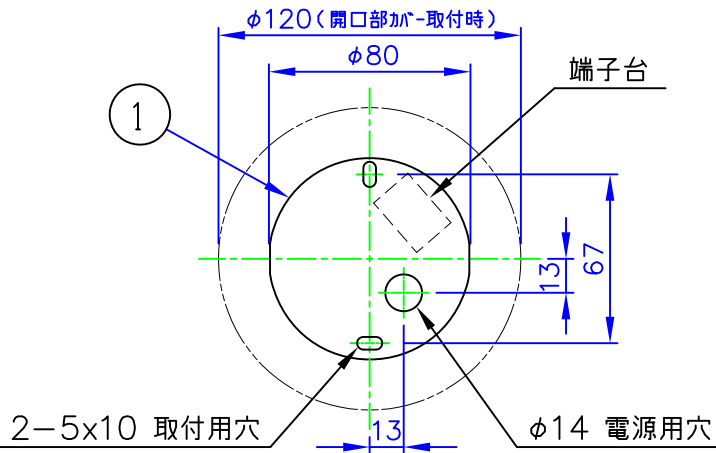
取付面図
