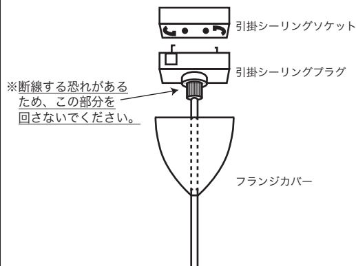
角型引掛シーリング
