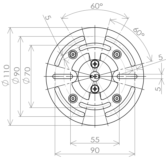
天井ブラケット詳細 尺度 1/2
